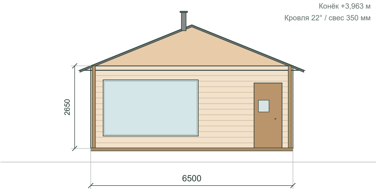
Главный фасад
