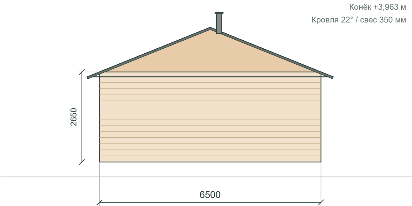
Задний фасад
