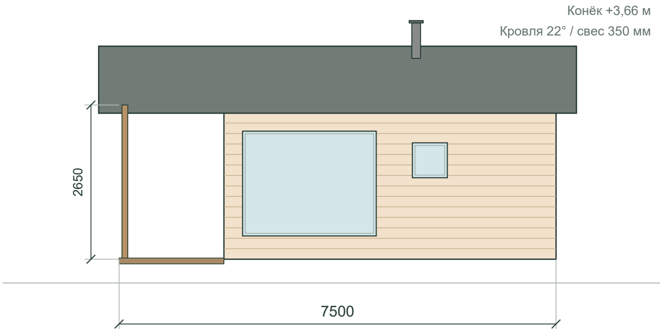
Правый фасад
