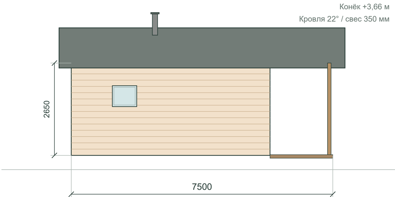
Левый фасад
