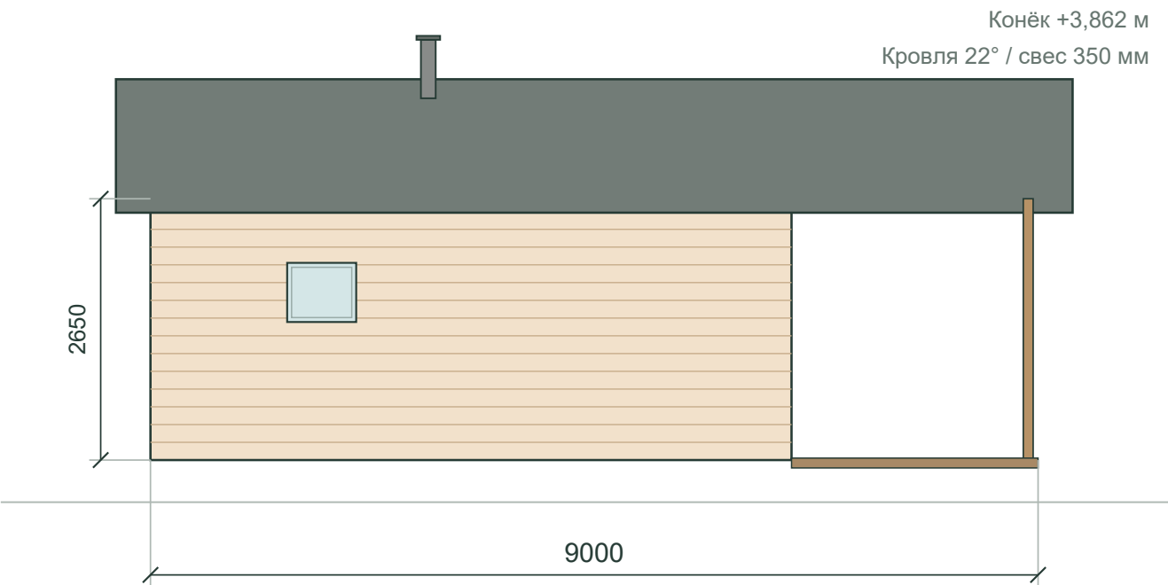
Левый фасад
