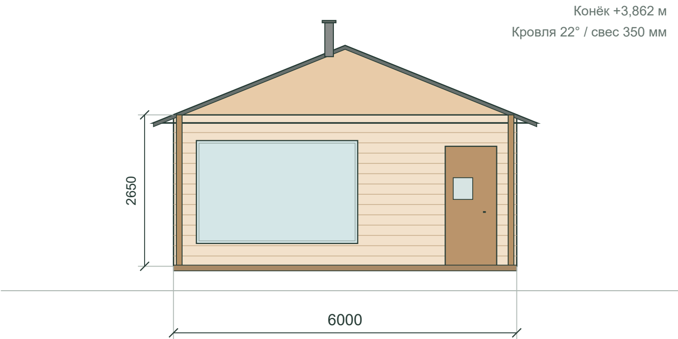
Главный фасад
