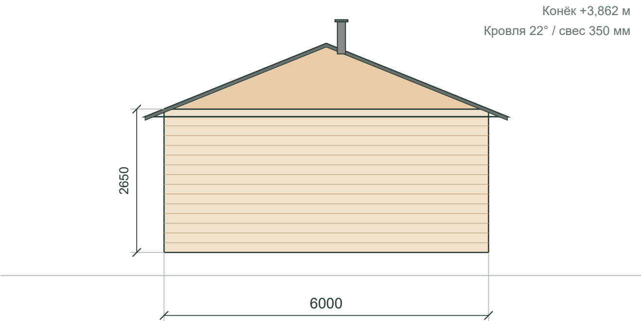
Задний фасад
