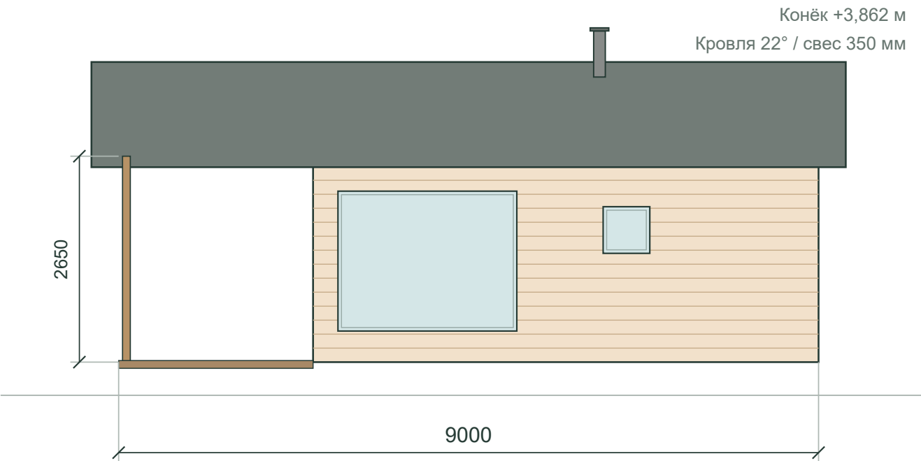
Правый фасад
