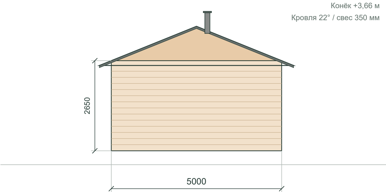
Задний фасад
