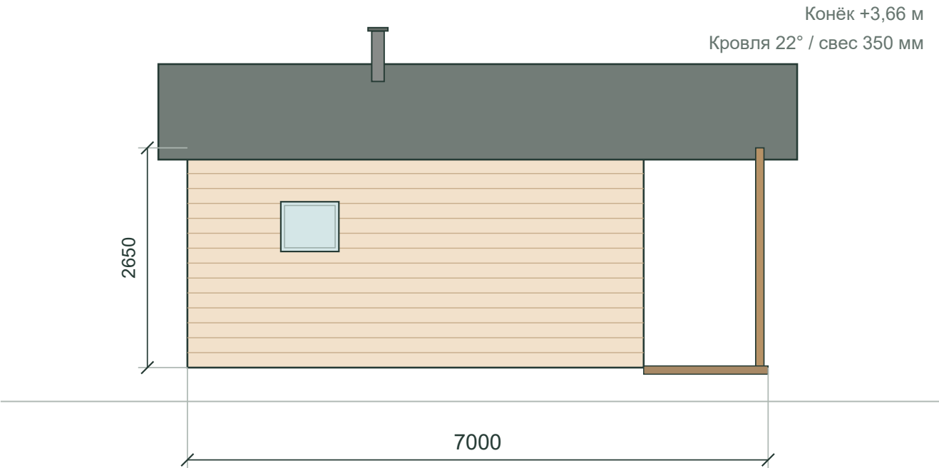
Левый фасад
